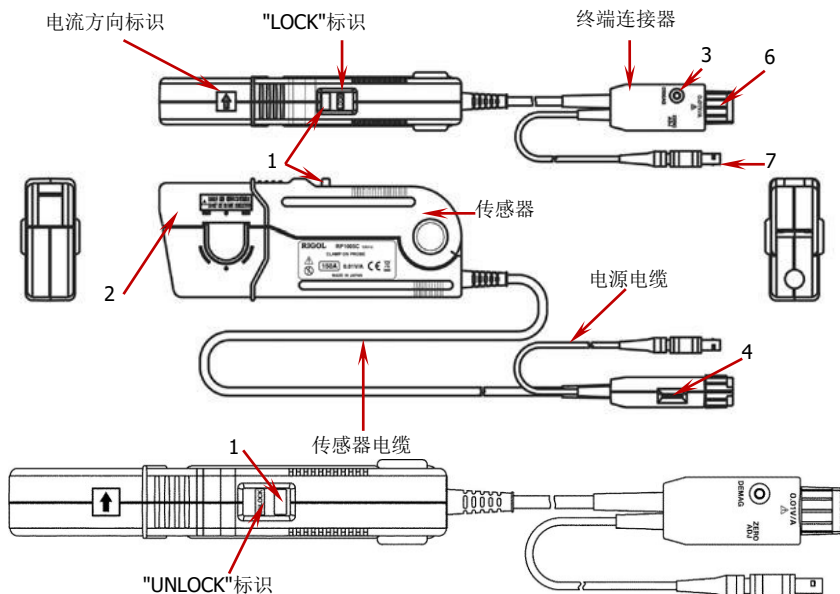
图 2 RP1005C/RP1006C 部件示意图
